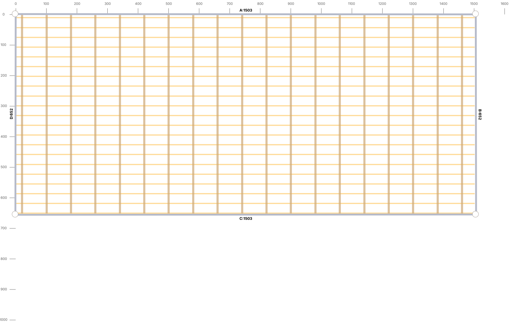
Dachbemaßung Dachfläche 2
