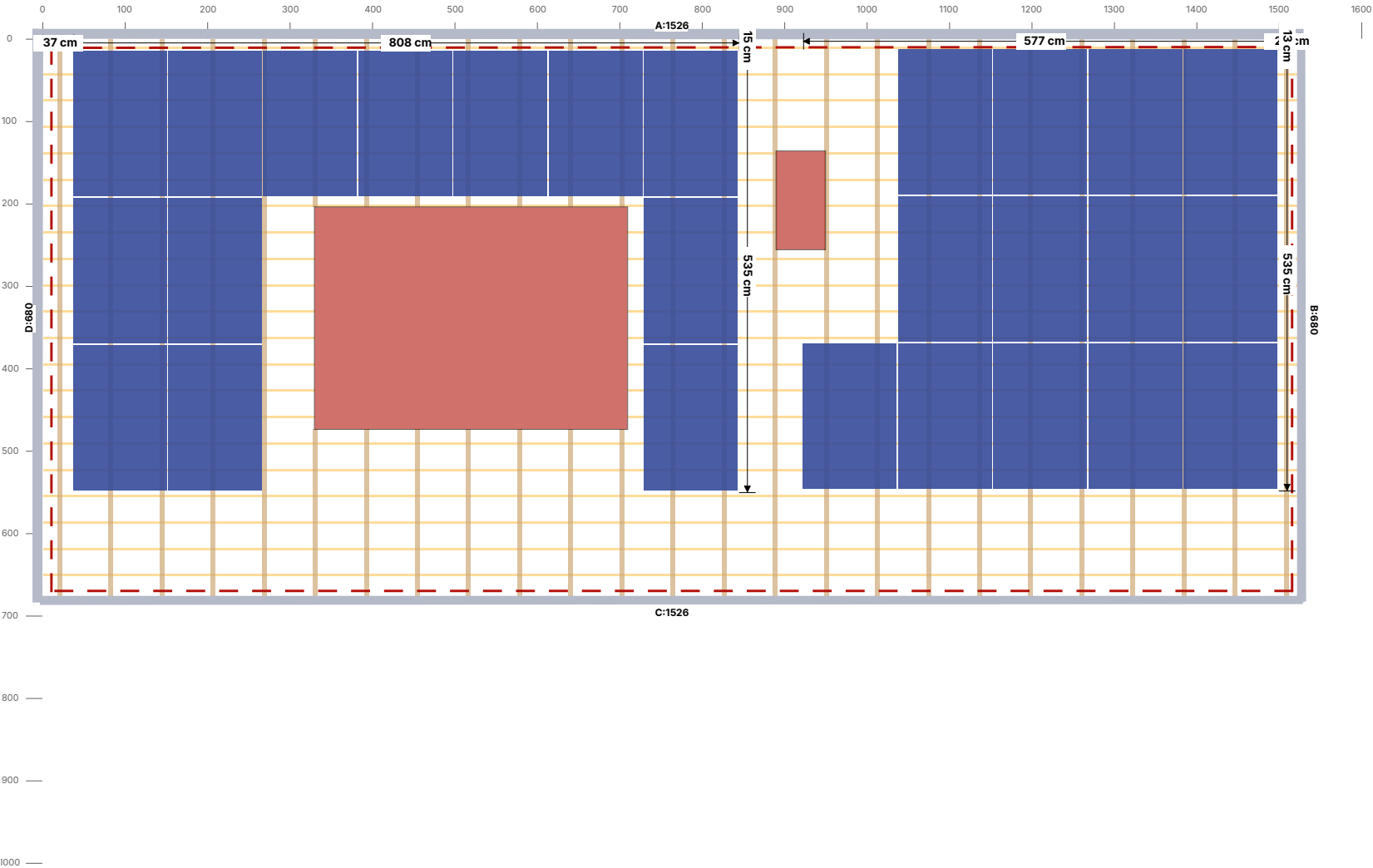
PV-Generator Dachfläche 1
