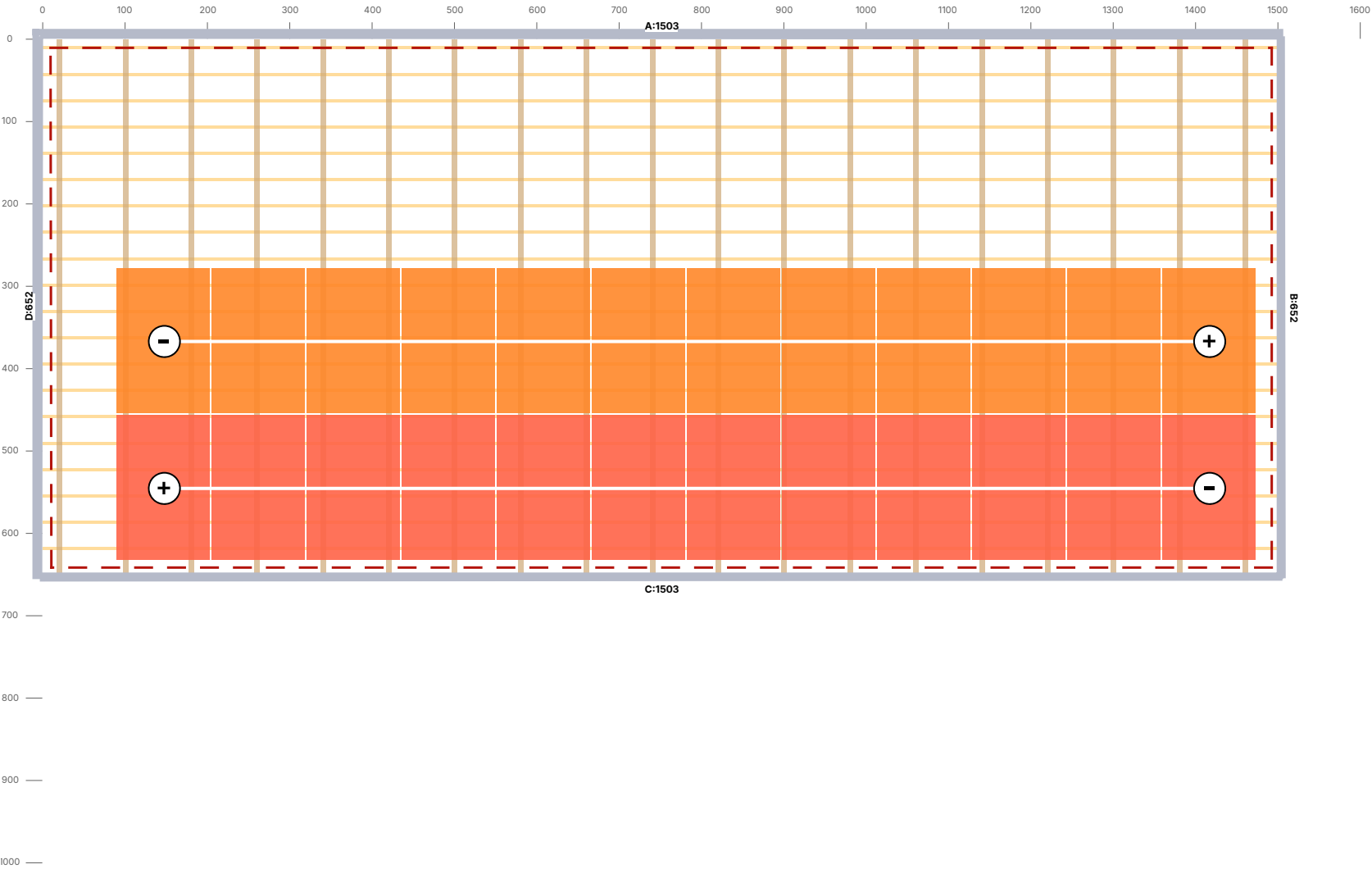
Verstringung Dachfläche 2
